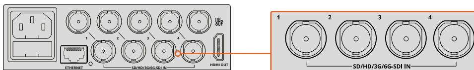
Conecte las fuentes a las entradas SDI.
